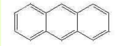
Obrázek 1: Molekula anthracenu
