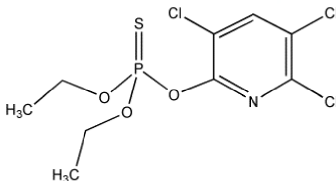
Obrázek 1: Struktura chlorpyrifosu
