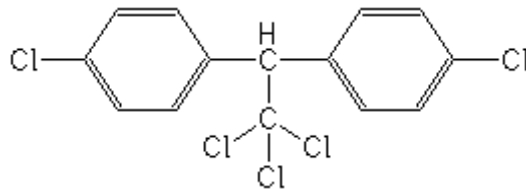
Obr. 1. Molekula DDT
