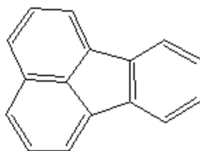
Obrázek 1: Struktura fluoranthenu
