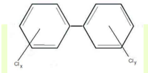
Obrázek 1: Obecná struktura molekuly PCB. Jednotlivé kongenery se liší stupněm chlorace a polohou atomů chloru na aromatických jádrech.
