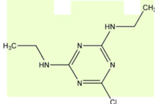
Obrázek 1: Struktura simazinu
